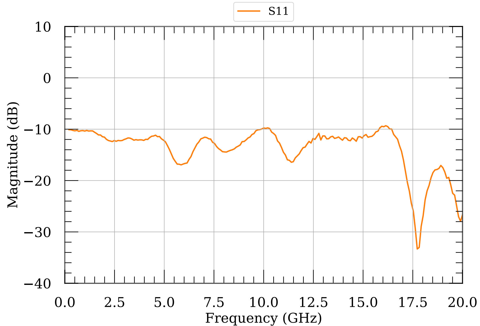
LNA S-params module078v2
